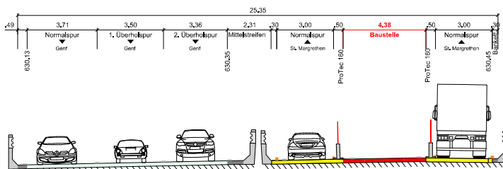
Sitterviadukt-Kreuzbleiche: Beispiel einer Verkehrsführung mit Spurabbau
